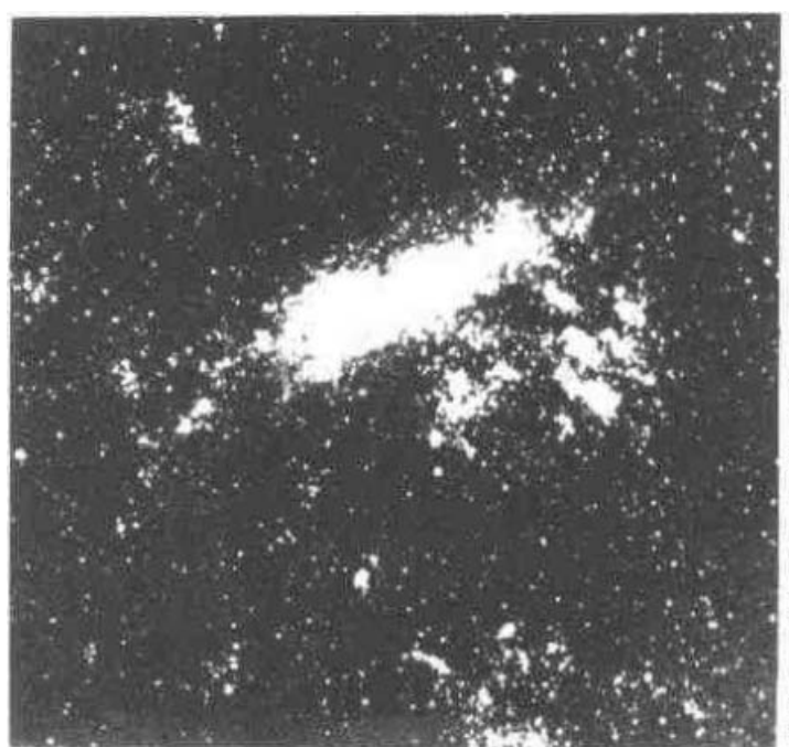
图 9.20 大麦哲伦云
