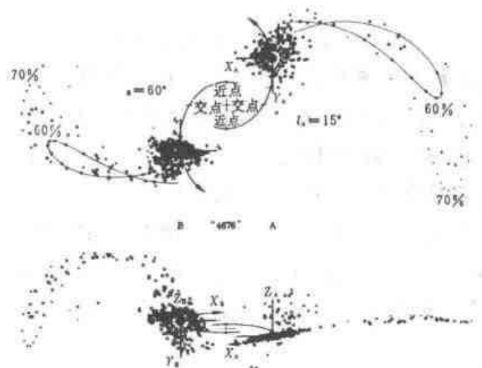
图 9.46 数值模拟两星系相碰形成尾巴
