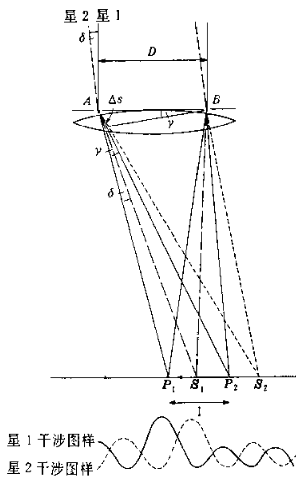
图 3.30 迈克耳孙干涉仪光线的示意图
