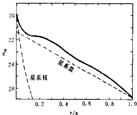
图 9.16(A) 每平方角秒的照相星等与 \frac{r}{a}
