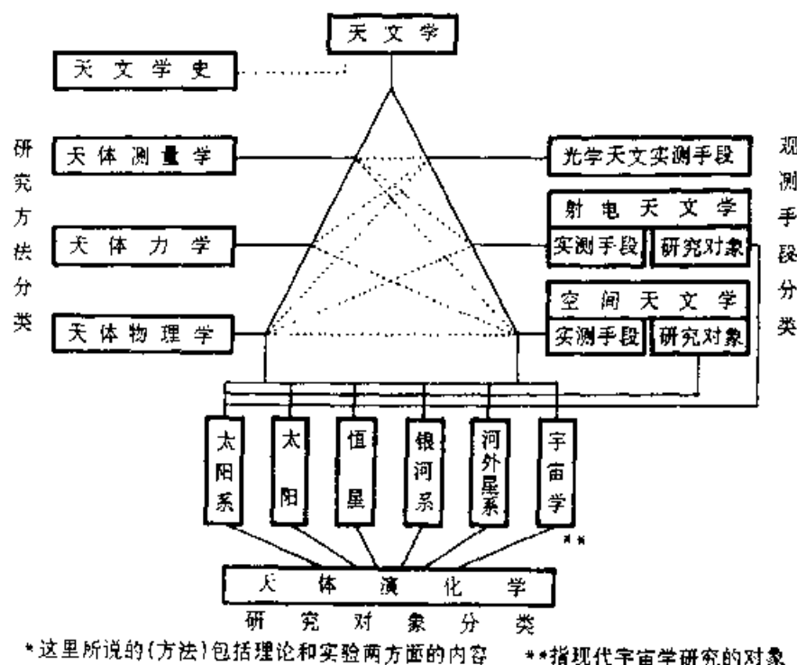
图 1.6 天体物理学关系图
