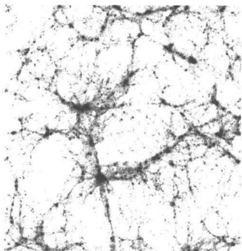
图 10.22 结构形成的数值模拟(取自室女团研究组 1998)宇宙模型为 \Lambda CDM, 粒子数为 256^3 , \Omega_m = 0.3 . 每边尺度为 240h^{-1}\text{Mpc} .
